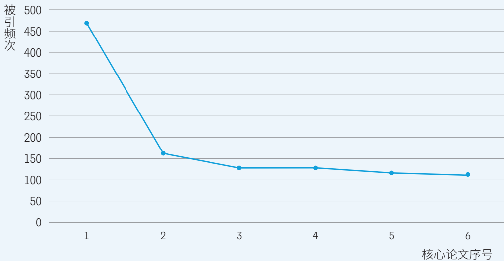
图 24 “脉冲星计时阵列探测纳赫兹引力波”研究前沿中核心论文的被引频次分布曲线
